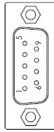
VIEW A-A
